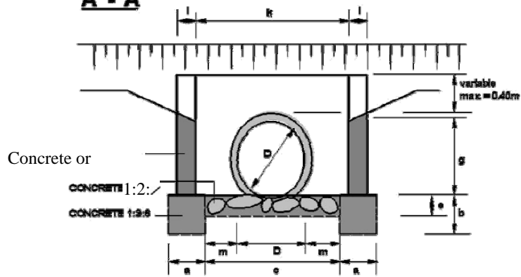
A - A
